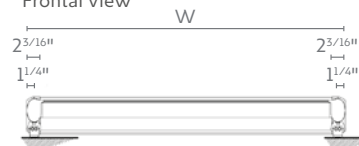
Single module
