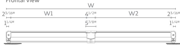
Double module
