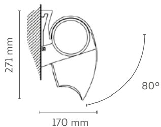
80° Montaje a pared
