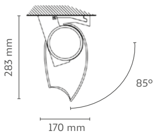
85° Montaje a techo
