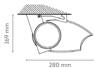
Montaje a techo
