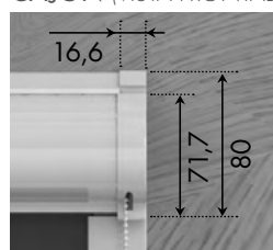
CAJÓN (VISTA FRONTAL)
