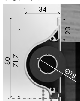
CAJÓN (VISTA LATERAL)
