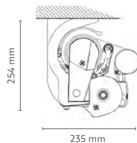
Montaje a techo con soporte universal
