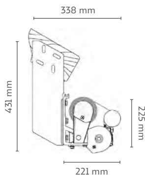
Instalación bajo cubierta
