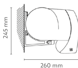
Montaje a pared con terminal cofre
