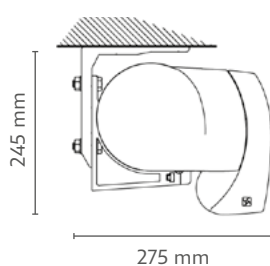
Montaje a techo con terminal cofre
