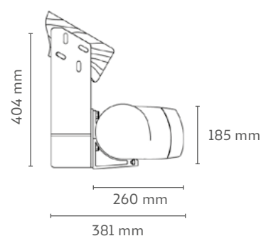
Instalación entre paredes
