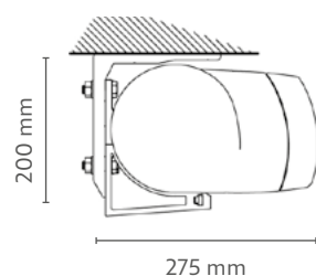
Montaje a techo
