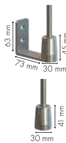
GUÍA VARILLA INOX Ø10 mm
