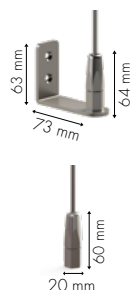
GUÍA CABLE INOX Ø5 mm
