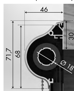
Cassonetto (vista laterale)
