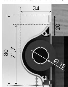
Cassonetto (vista laterale)
