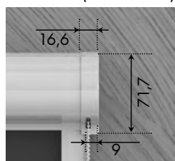
Cassonetto (vista frontale)
