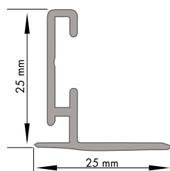
GUIDA LATERALE "L" 90 Y 60 (OPTIONAL S1)
