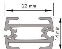
PROFILO INTERMEDIO (UNIONE TESSUTI)
