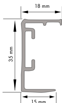
GUIDA LATERALE "U" (OPTIONAL S3)
