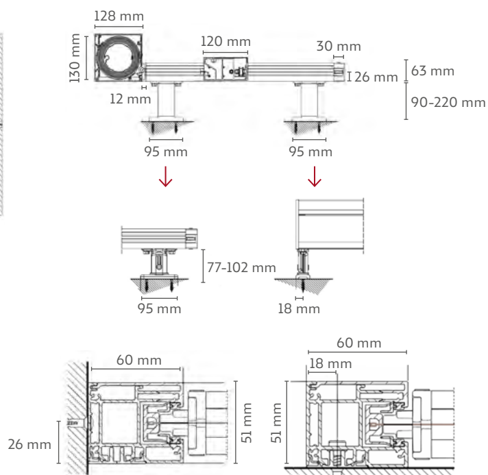
Vista laterale
