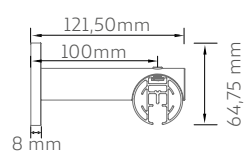
Binario Aeris a parete
