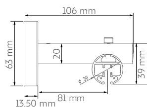
Binario Elpis a parete
