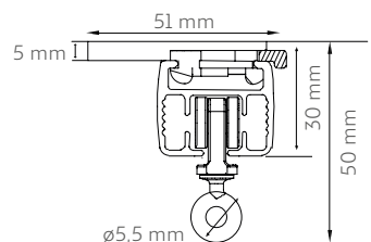
Binario Glydea soffitto
