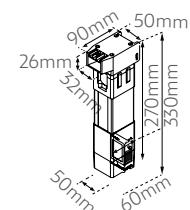
Motore binario XXL a soffitto pe LYNX
