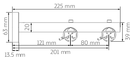
Binario Elpis doppio
