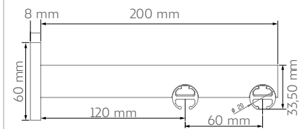
Binario Dike doppio
