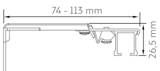
Onde Perfette asta a soffitto
