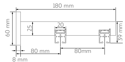
Binario Kali doppio
