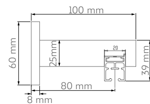
Binario Kali a parete
