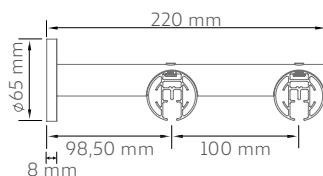
Binario Aeris doppio
