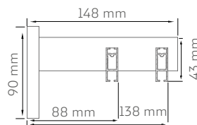
Binario Urban a soffitto
