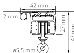
Rail Glydea rotatif au plafond
