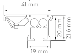
Ondulations Parfaites baston façade
