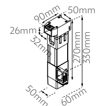
Moteur Rail XXL plafond pour LYNX
