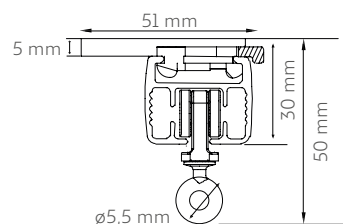
Rail Glydea plafond
