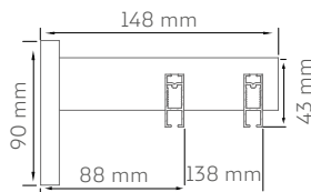
Rail Urban plafond
