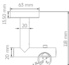
Rail Elpis plafond
