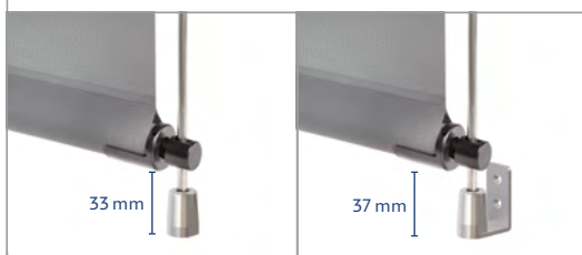
Guidage par tige INOX ø10 mm
