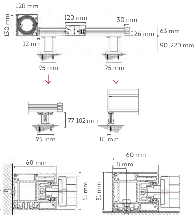
Módulos y guías
